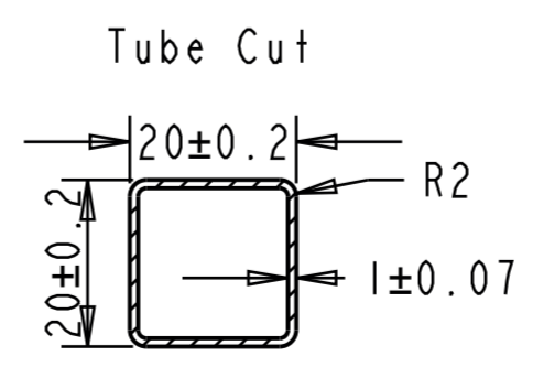
SECTION A-A SCALE 1.000
